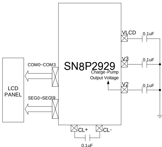
1/3 偏压, C 型 LCD 应用电路
