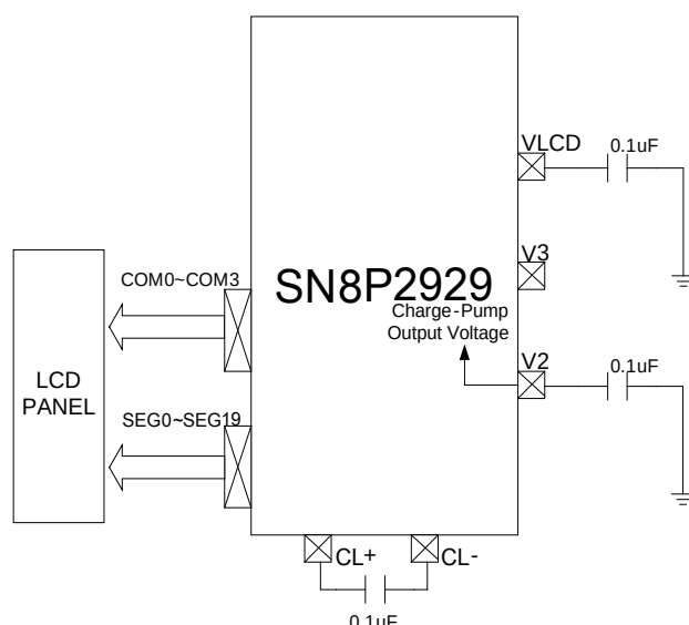
1/2 偏压, C 型 LCD 应用电路
