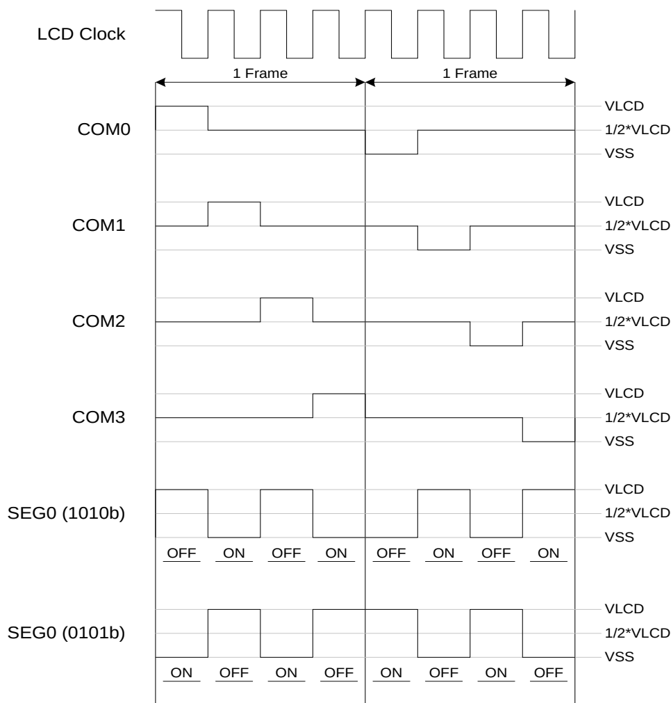
LCD 驱动波形，1/4 duty, 1/2 bias
