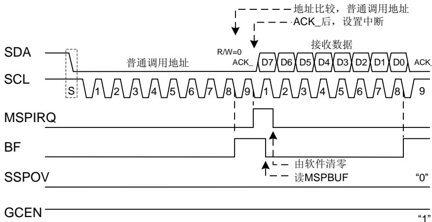
通用地址应答时序图
