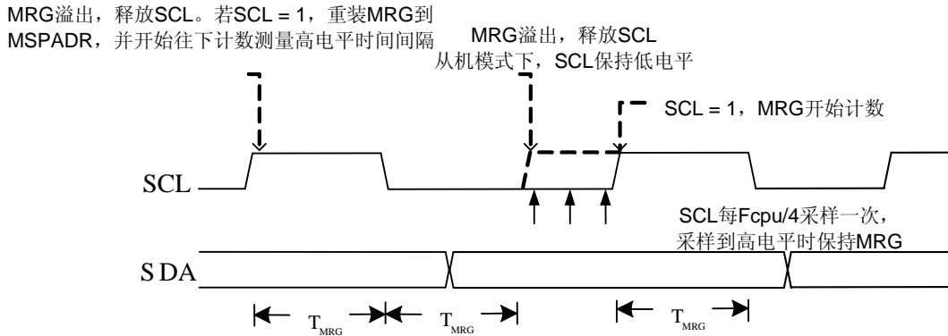
时钟仲裁流程时序示意图
