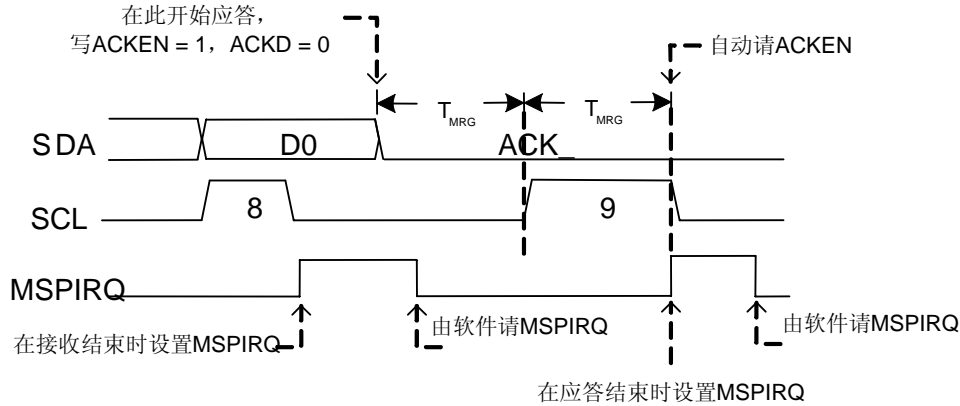
应答流程时序示意图
