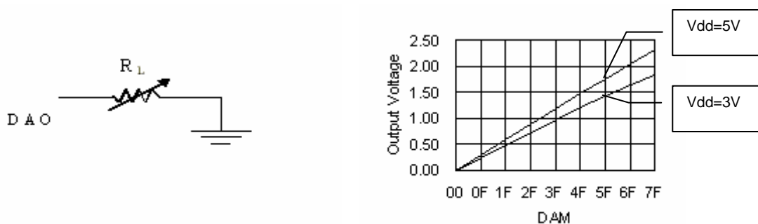
带 R_L 的 DAO 电路
