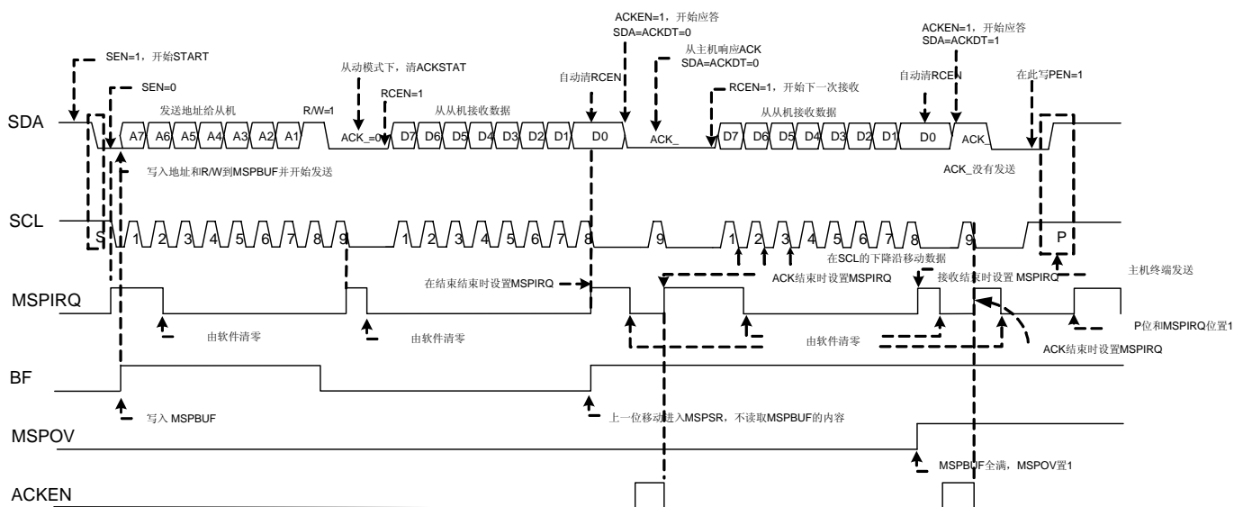
MSP 主机接收模式时序示意图
