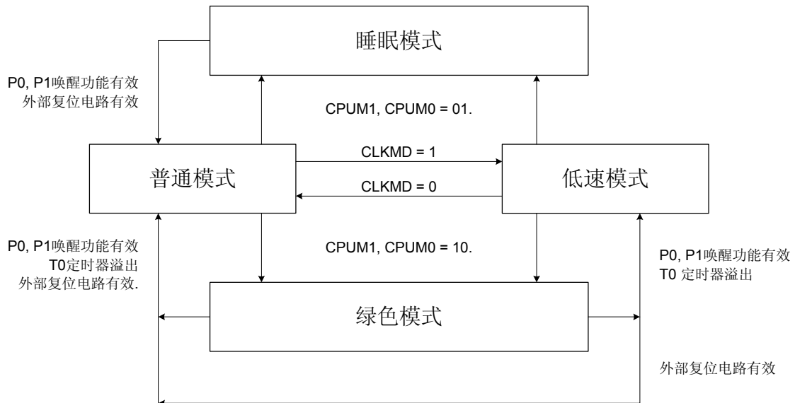
系统模式切换框图
